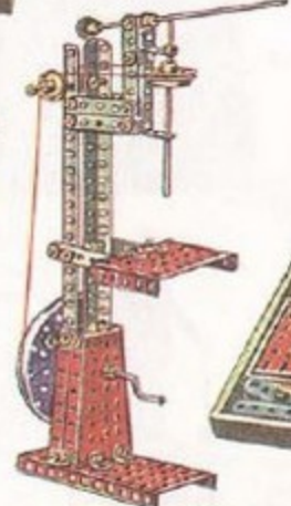
Bohrmaschine gebaut mit Kasten Nr. 3 F
