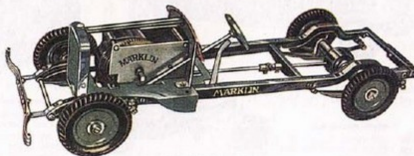
Chassis (Fahrgestell)
