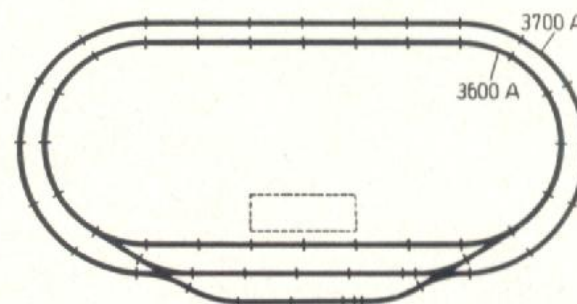
Fig. B 3600/621 • Ovalo de doble vía con estación de paso • Tamaño 200X105 cm. • Piezas de vía B 3600, 11 A, 1 AA, 24 D, 2 D 1/4 , 1 D 1/8 • 1 par de desvíos MWS, dos transversales de unión doble DKWS y además 12 piezas de vía 3700 A 1/1
